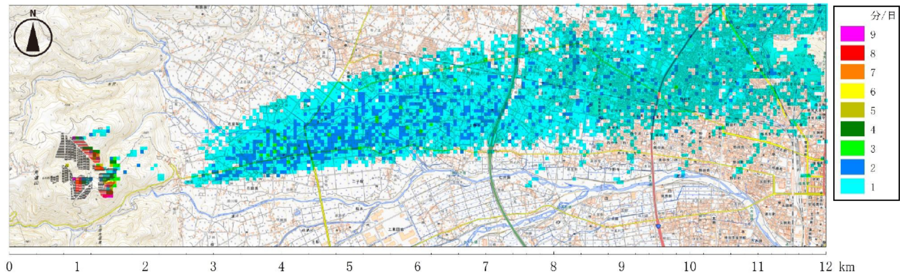
図 6-1(2) 反射光影響範囲図 (春分の日の前後 10 日間 (2025 年 3 月 10~30 日) の最大日の時間数)
